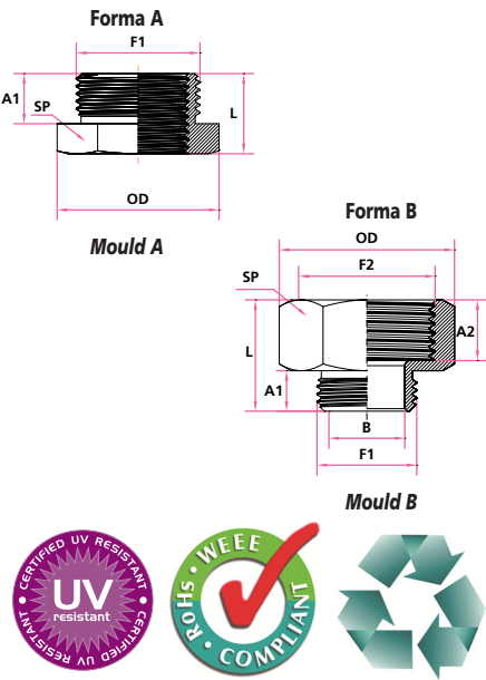
RGG - Riduzioni esagonali filetto maschio GAS - filetto femmina GAS
